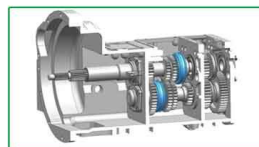
Cambio de lanzadera 12F+12R
